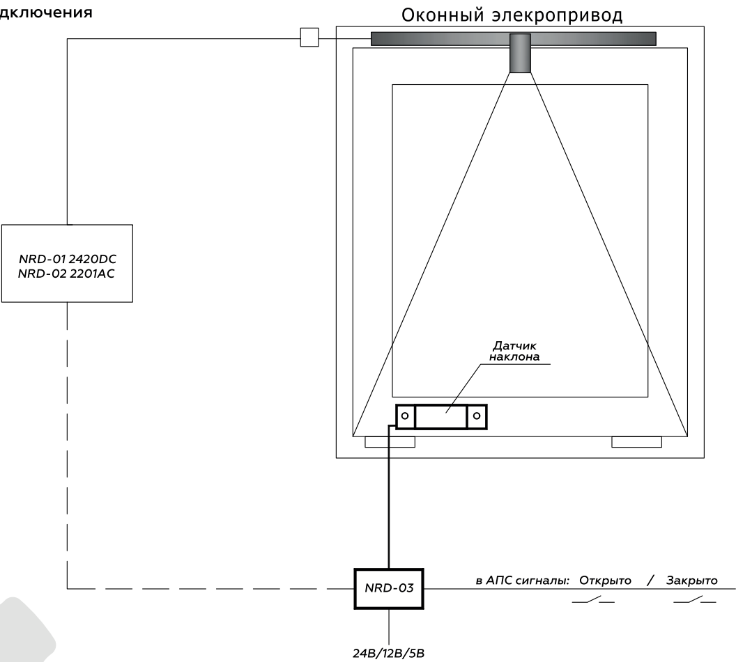
Схема подключения
