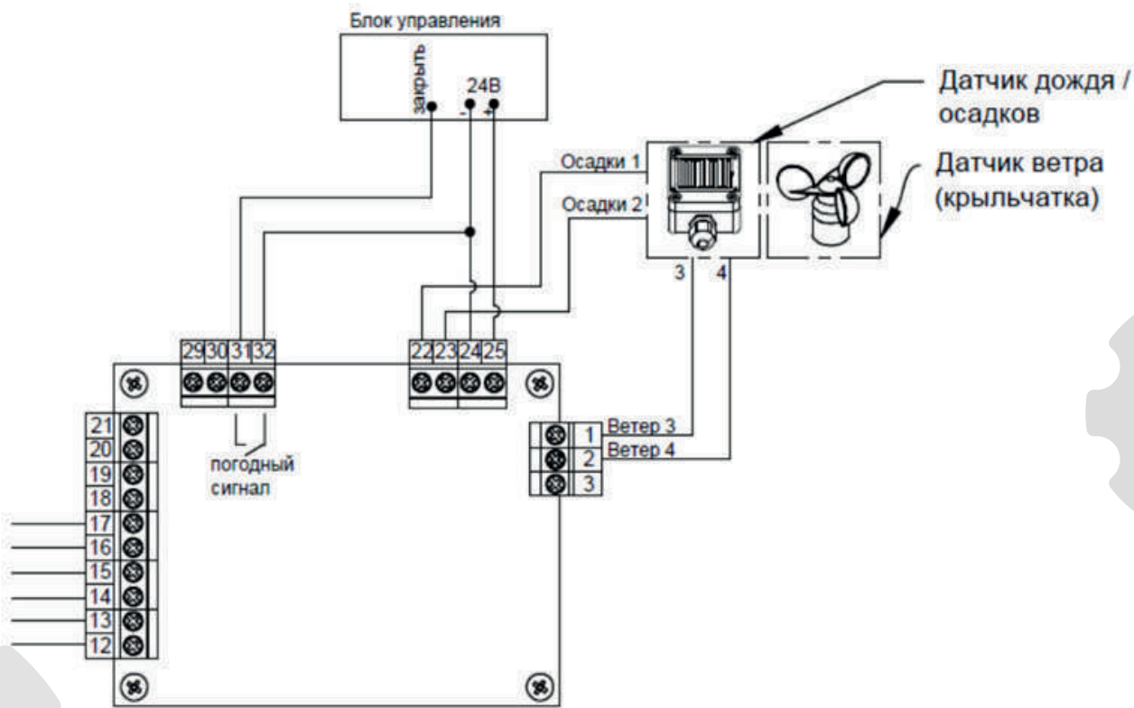
Схема подключения метеостанции
