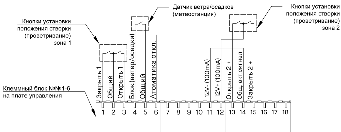
Рис. 7. Схема подключения кнопок установки положения (проветривания) и датчиков ветра/осадков (метеостанции)
