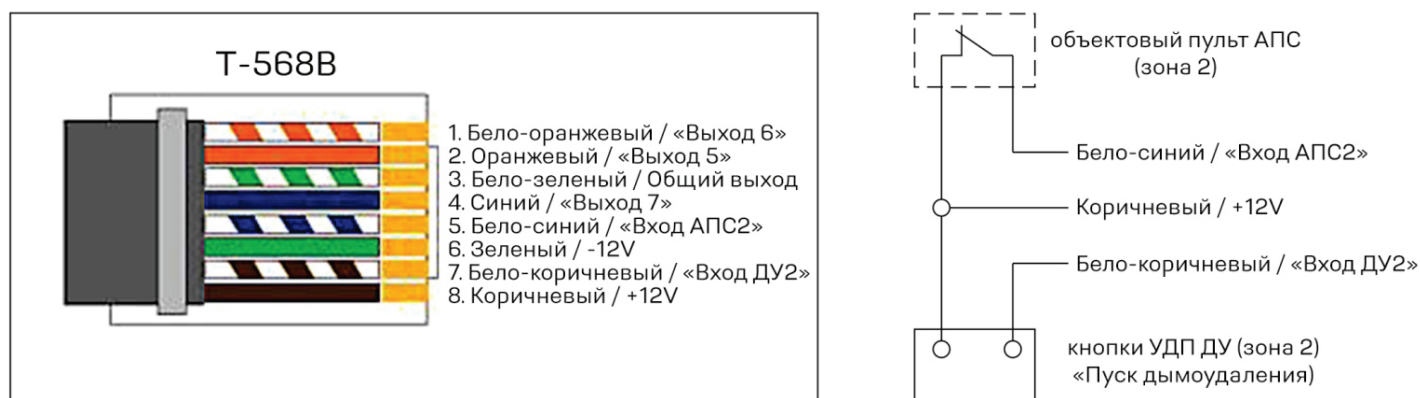
Рис. 5.1. Схема подключения сигналов АПС и УДП ДУ для зоны 2.
