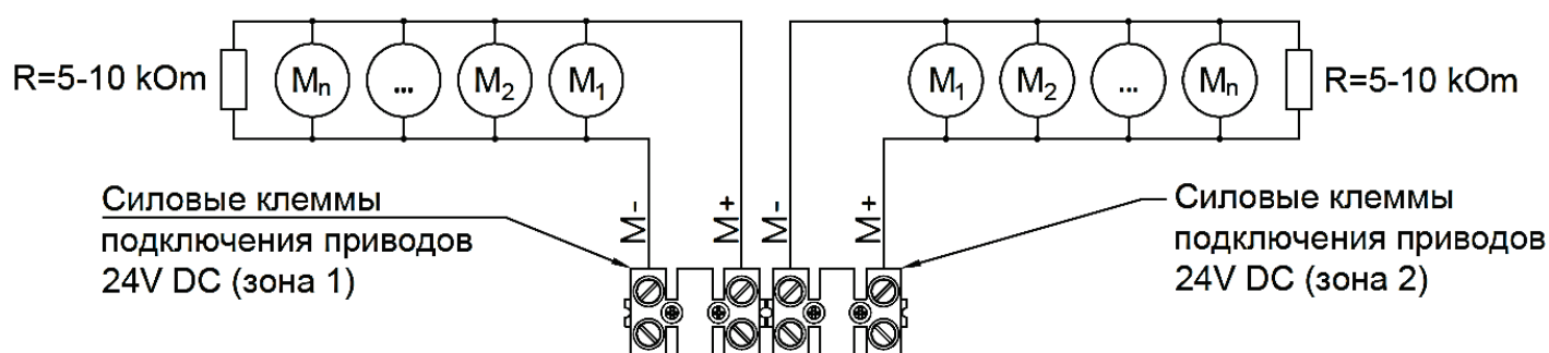
Рис. 4. Схема подключения приводов 24V DC
