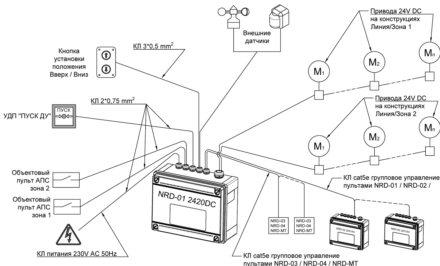
Рис. 3. Схема прокладки кабельных линий
