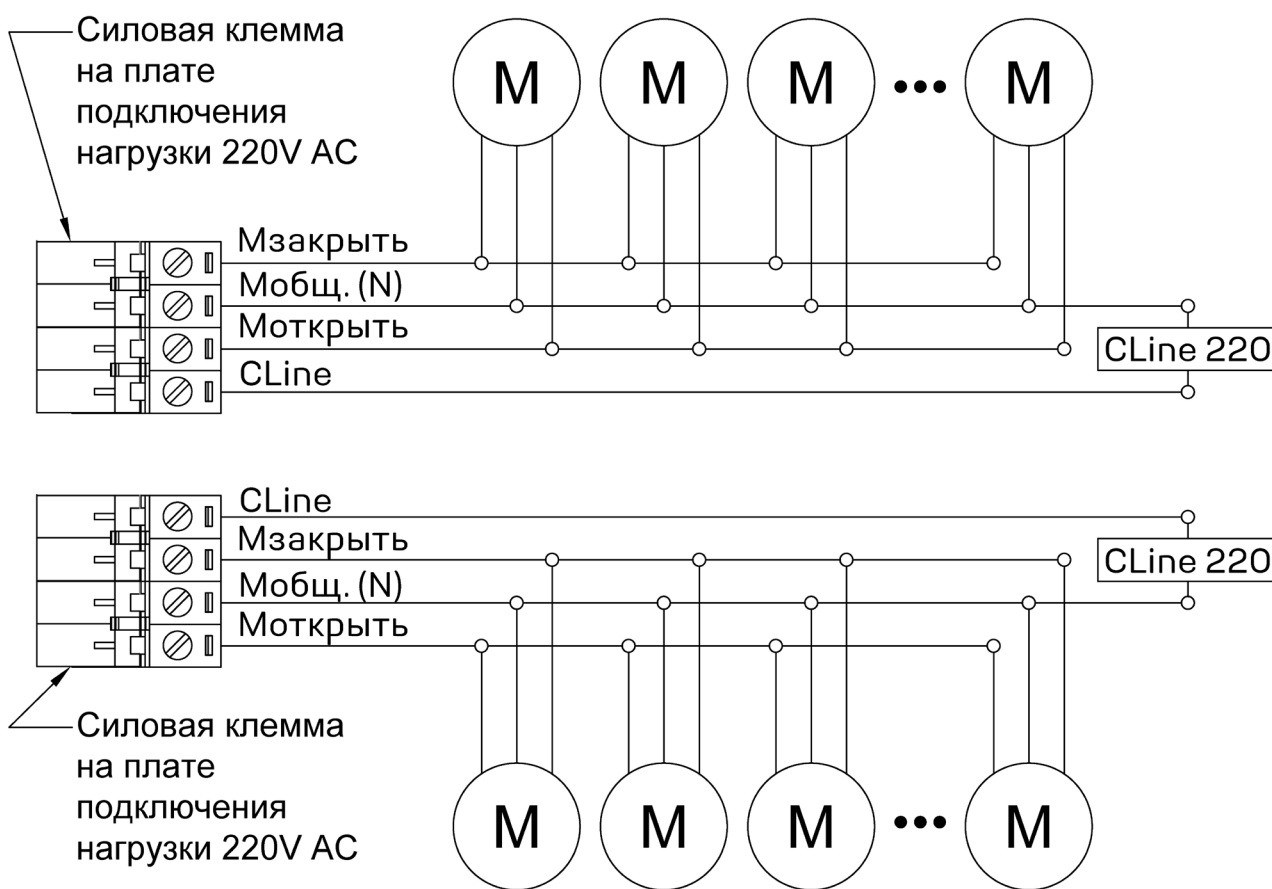
Рис. 4. Схема подключения привода 220V AC
