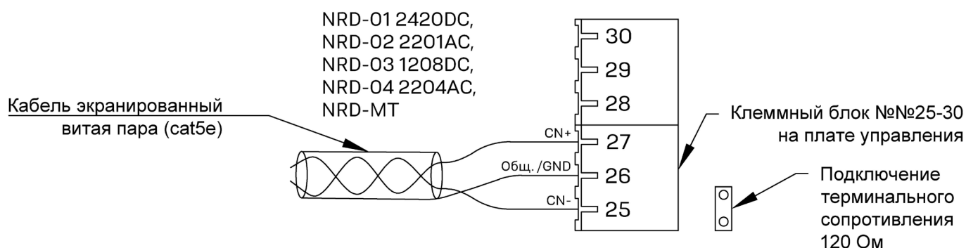
Рис. 8. Схема подключения коммуникационной шины (групповое управление).
