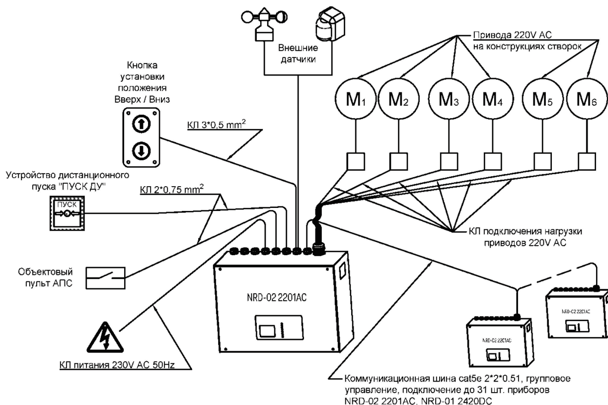
Рис. 3. Схема прокладки кабельных линий
